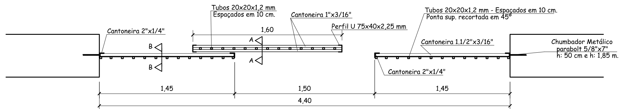
Planta Baixa
